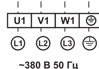
Схема подключения вентиляторов ВРС-К мощностью свыше 2,2 кВт
