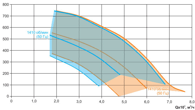
RW-LZ/LT-90-50-A.F.ПЦ.45.2,2.4
