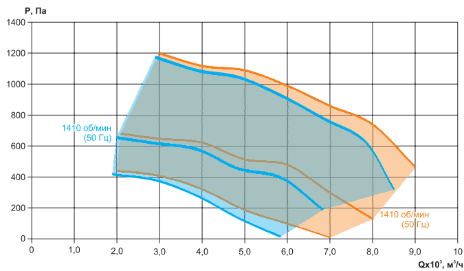
RW-LZ/LT-100-50-A.F.ПЦ.50.3.4
