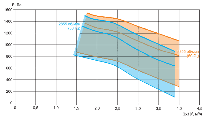
RW-LZ/LT-60-35-A.F.ПЦ.35.2,2.2
