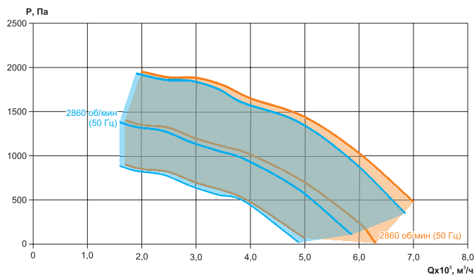
RW-LZ/LT-80-50-A.F.ПЦ.35.3.2
