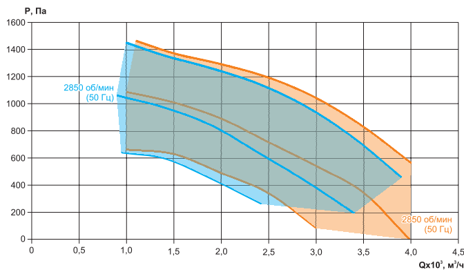
RW-LZ/LT-60-35-A.F.ПЦ.31.1,5.2
