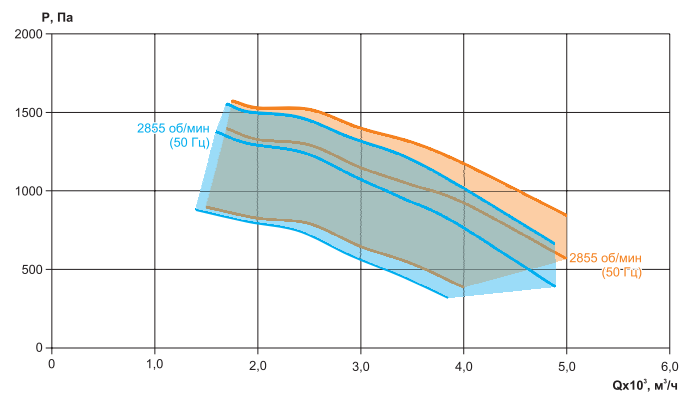
RW-LZ/LT-70-40-A.F.ПЦ.35.2,2.2
