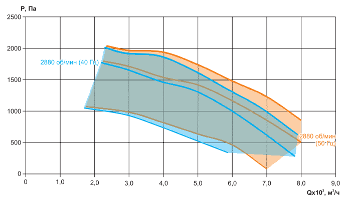
RW-LZ/LT-80-50-A.F.ПЦ.40.4.2
