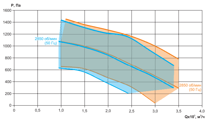
RW-LZ/LT-60-30-A.F.ПЦ.31.1,5.2
