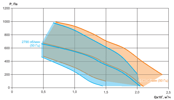
RW-LZ/LT-50-25-A.F.ПЦ.25.0,55.2
